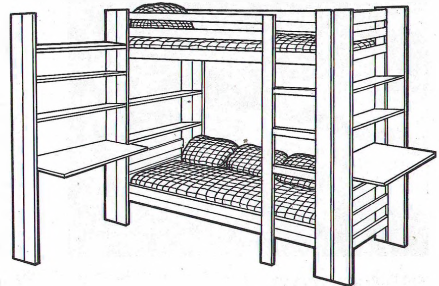
Рис. 2. Блок детской мебели с двумя спальными и двумя рабочими местами, с открытыми полками
