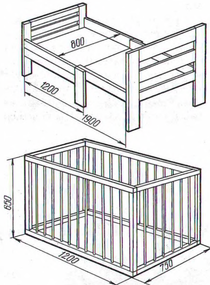
Рис. 1. Кровать с изменяемой длиной со съемным манежем
