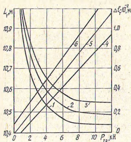
Рис. 3. Графики изменения длины L_T и деформации \Delta L_T = L_T - L_T^0 тросов управления от усилий в тросах ( q = 12,2 Н/м; F_T = 124,7 мм 2 ): 1, 4 — изменение длины и деформации тросов управления при базе лесовозного автопоезда 9 м; 2, 5 — при базе 10 м; 3, 6 — при базе 11 м
