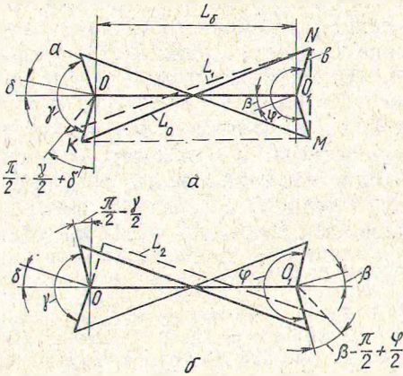
Рис. 1. Расчетная схема определения кинематических параметров сцепки: a — передаточного отношения; b — зоны неуправляемости
