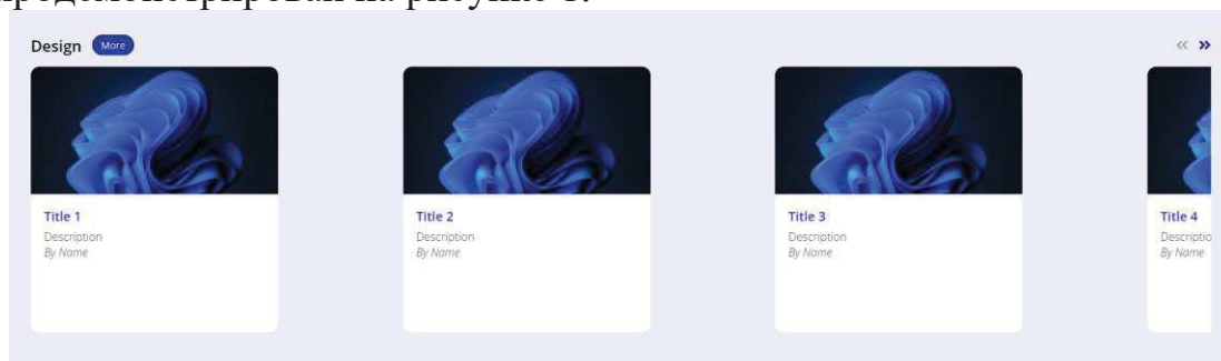
Рисунок 1 – СлайдерSwiper.js
