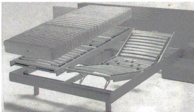
Рис. 1. Каркас кровати с регулируемым профилем основания из лат
