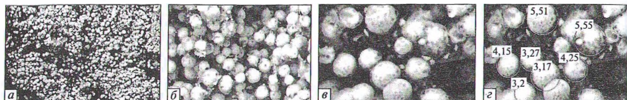
Рис. 2. Зольный остаток семян льна сорта McGregor в свете отраженных электронов. В золе сохранена сферическая структура глобидов. Диаметр глобидов (мкм) измерен с использованием программного обеспечения микроскопа JSM-5610 LV. Ув.: а – 500; б – 2000; в – 5000; г – 5000
