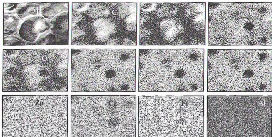
Рис. 3. Рентгенофлуоресцентные карты распределения элементов в клетках запасающей паренхимы семядолей льна сорта McGregor: I – нативное изображение клеток в режиме низкого вакуума. Темные точки на изображении
