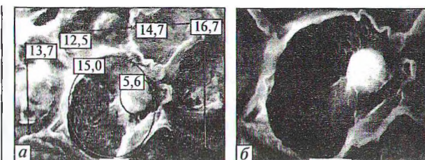
Рис. 1. Клетки запасающей паренхимы семядолей льна сорта McGregor в свете отраженных электронов. Фитиновый глобид — светлое сферическое образование справа по экватору клетки. Абсолютные размеры клеток и клеточных структур (мкм) указаны стрелками (измерения проведены при использовании программного обеспечения микроскопа JSM-5610 LV); Ув.: а — 3500, б — 5000
