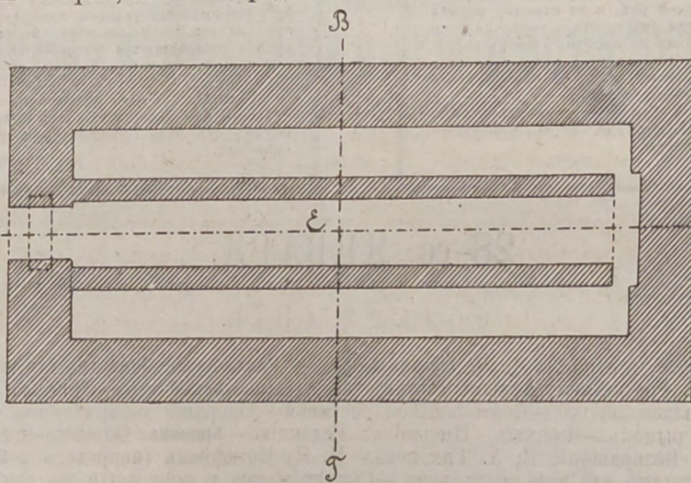
Рис. 1. Углеобжигательная печь А. П. Пятницкаго (планъ).
