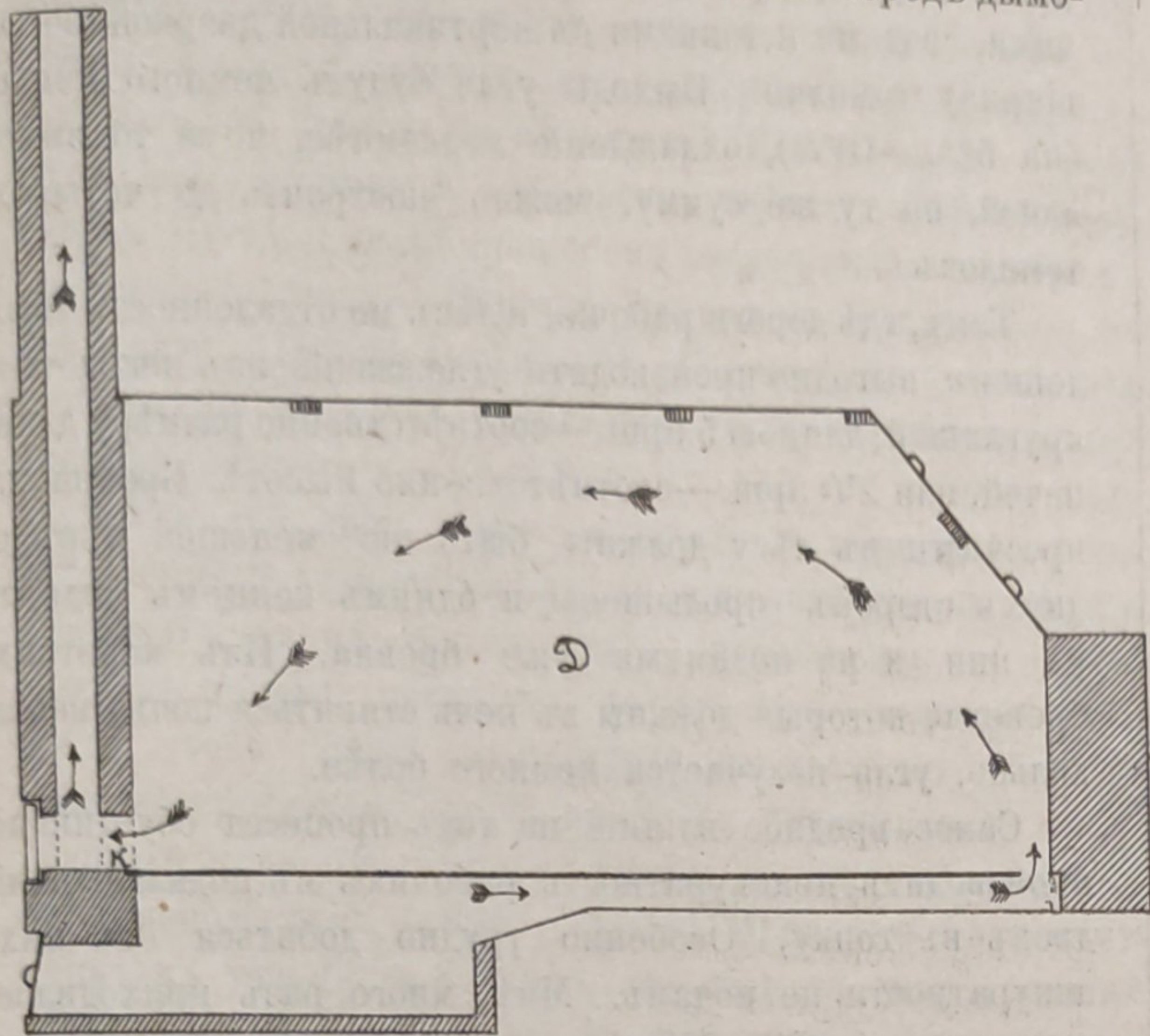
Рис. 2. Углеобжигательная печь А. П. Пятницкаго (разрѣзъ по АБ.)
