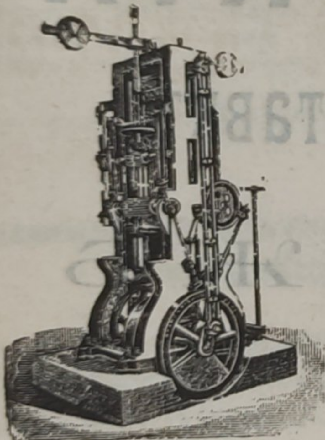
Постоянная лѣсопиливая рама.
