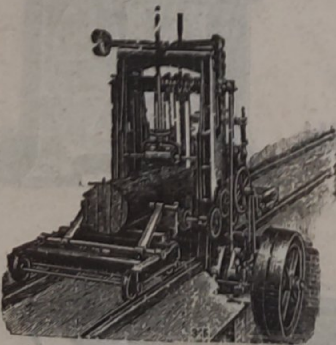
Переносная лѣсопилыная рама.
