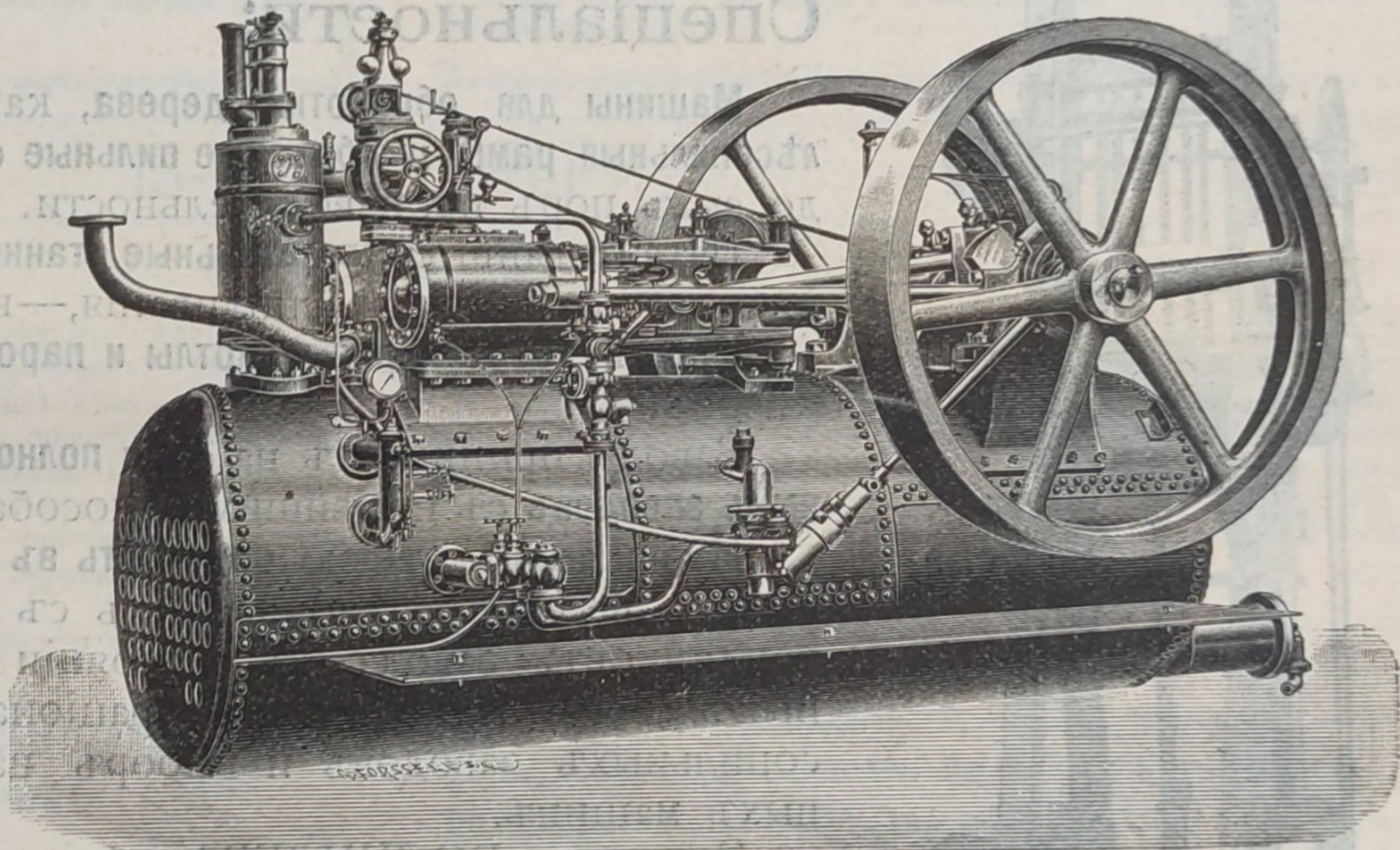
Локомобиль для лѣсопильнъ.
