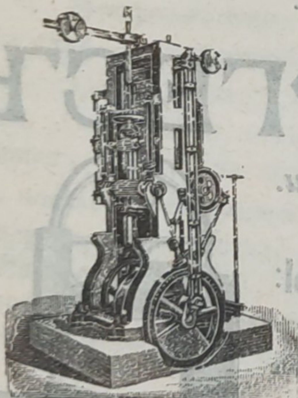
Постоянная лѣсопилыная рама.
