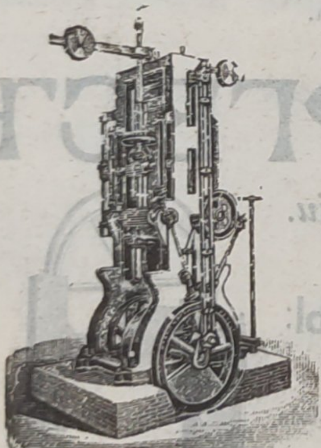
Постоянная лѣсопилная рама.
