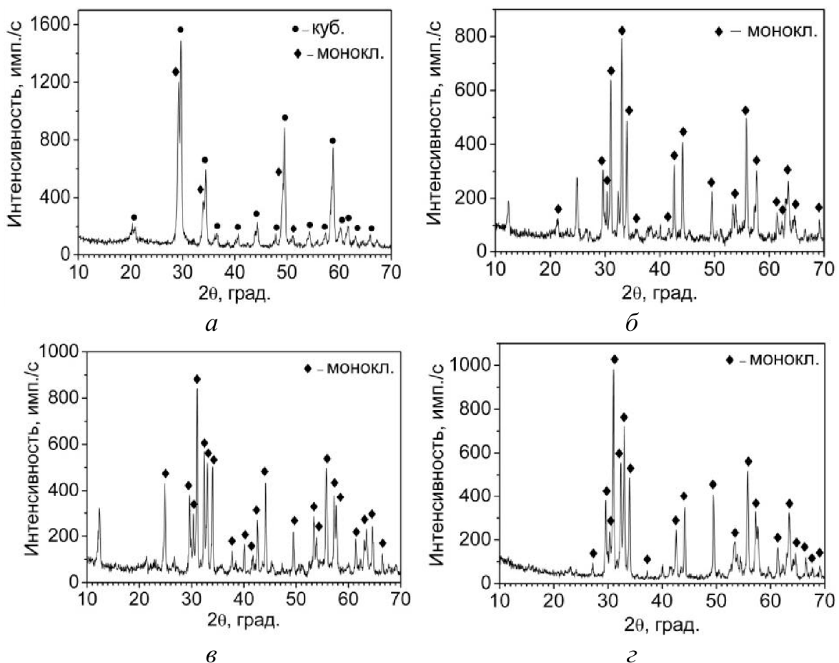
Рис. 2. Дифрактограммы исходной порошковой смеси ( а ) и образцов, спеченных при различной мощности W , кВт: б – 1,0; в – 1,2; г – 1,4
