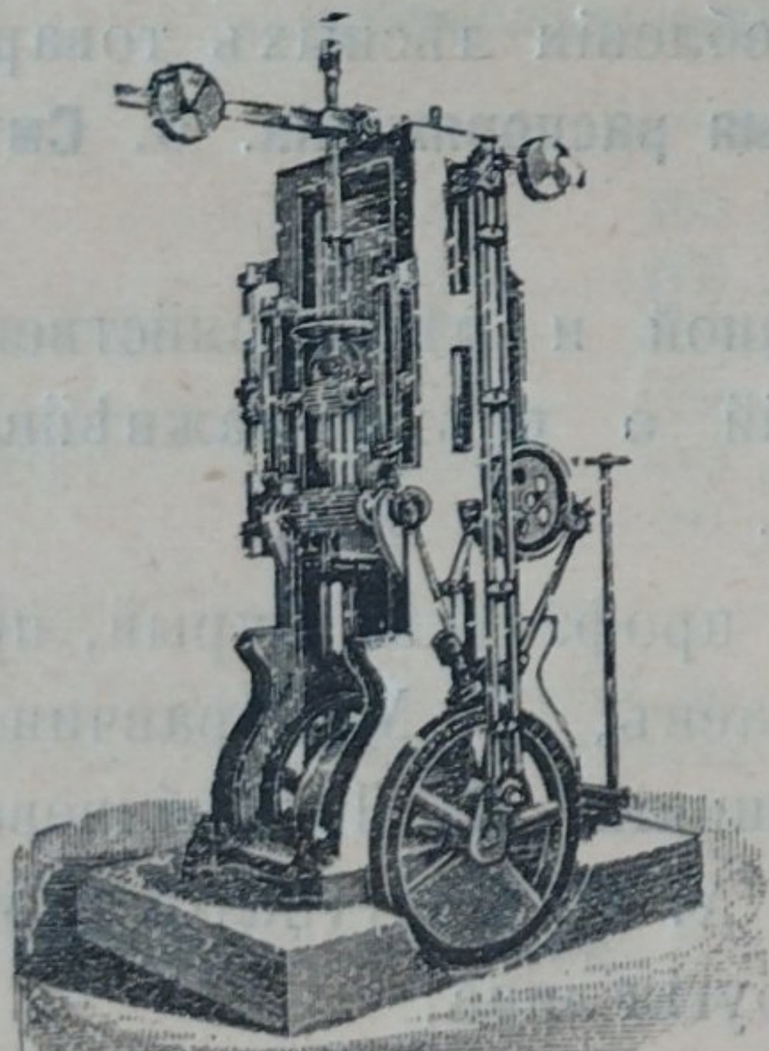
Постоянная лѣсопилная рама.
