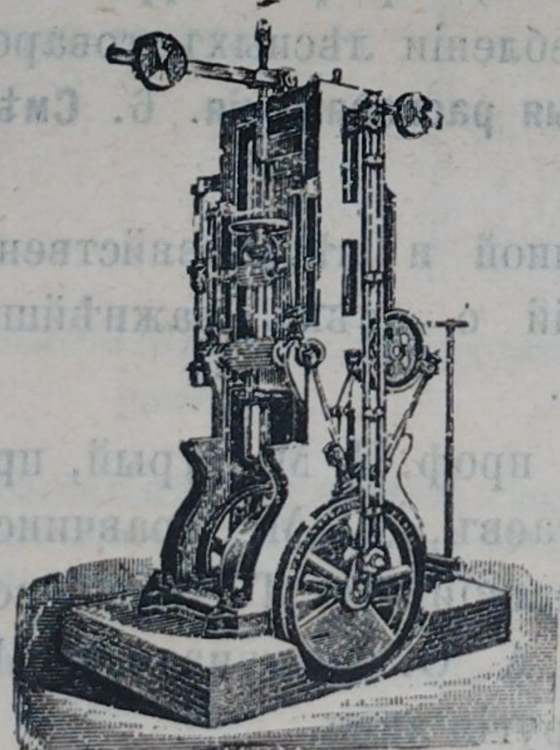
Постоянная лѣсопилная рама.
