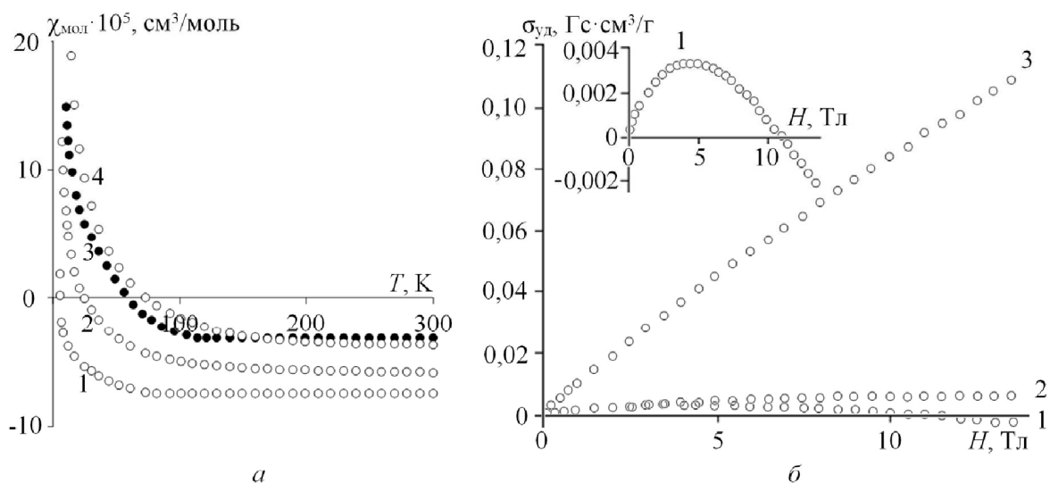
Рисунок 1. Температурные зависимости молярной магнитной восприимчивости ( \chi_{\text{мол}} ) индатов \text{La}_{1-x}\text{Pr}_x\text{InO}_3 с x = 0 (1), 0,001 (2), 0,003 (3), 0,004 (4) (а); полевые зависимости удельной намагниченности ( \sigma_{\text{уд}} ) при 5 К твердых растворов \text{La}_{1-x}\text{Eu}_x\text{InO}_3 ( x = 0,005 (1); 0,01 (2); 0,1 (3)) (б)
