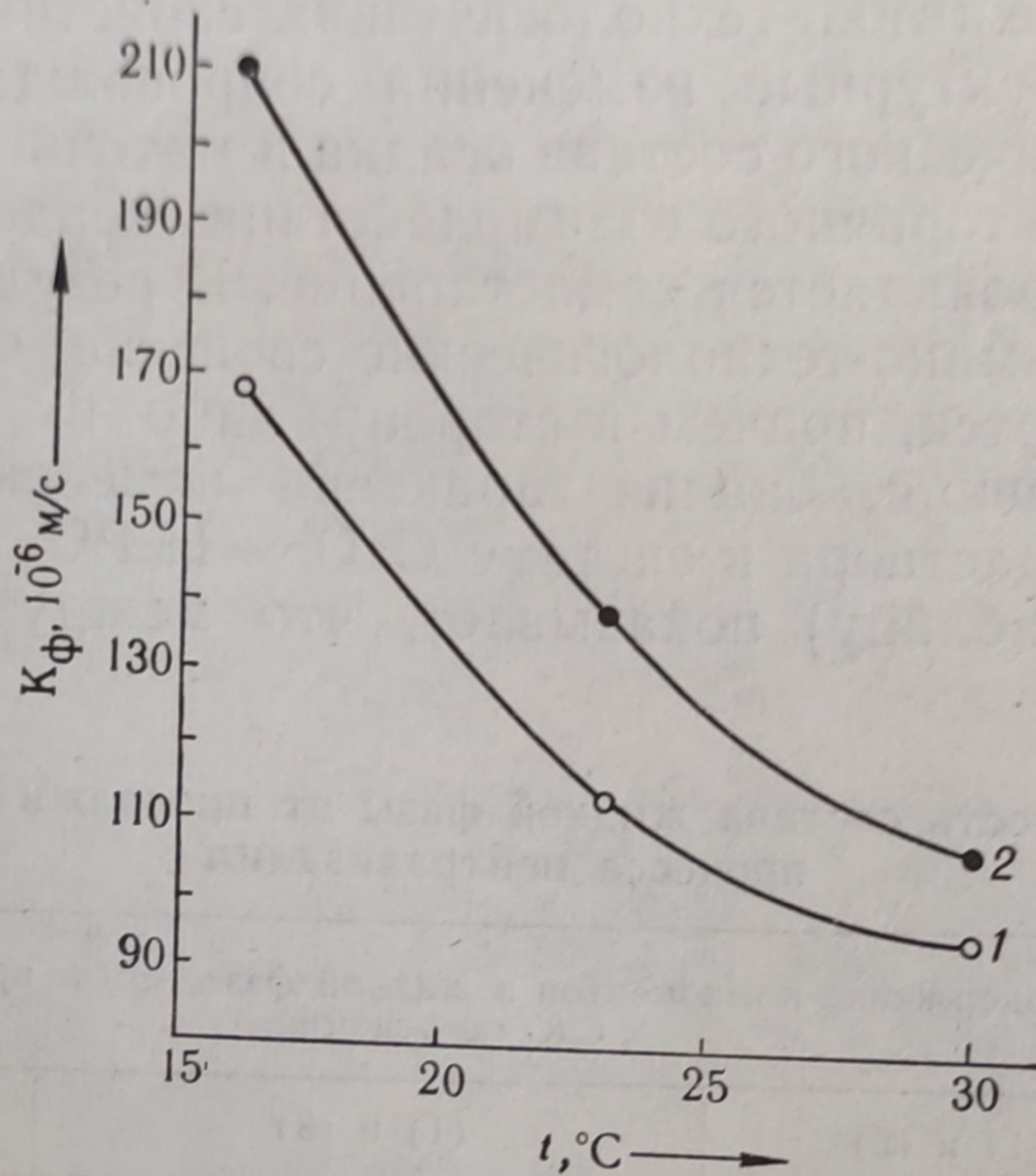
Рис. 2. Зависимость коэффициента фильтрации осадка от температуры процесса: 1 — продолжительность нейтрализации 30 мин; 2 — продолжительность нейтрализации 15 мин
