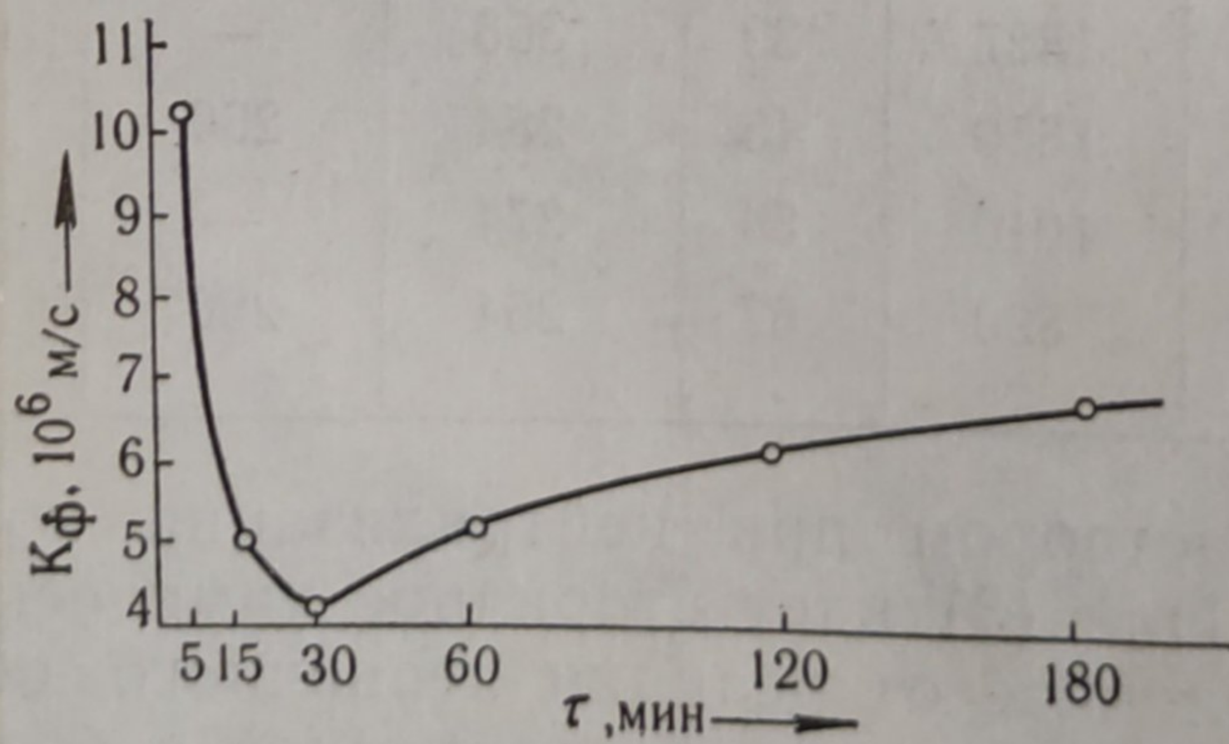
Рис. 3. Зависимость коэффициента фильтрации от продолжительности процесса нейтрализации. Введено стехиометрическое количество оксида кальция, рассчитанное по реакциям (1) и (4)
