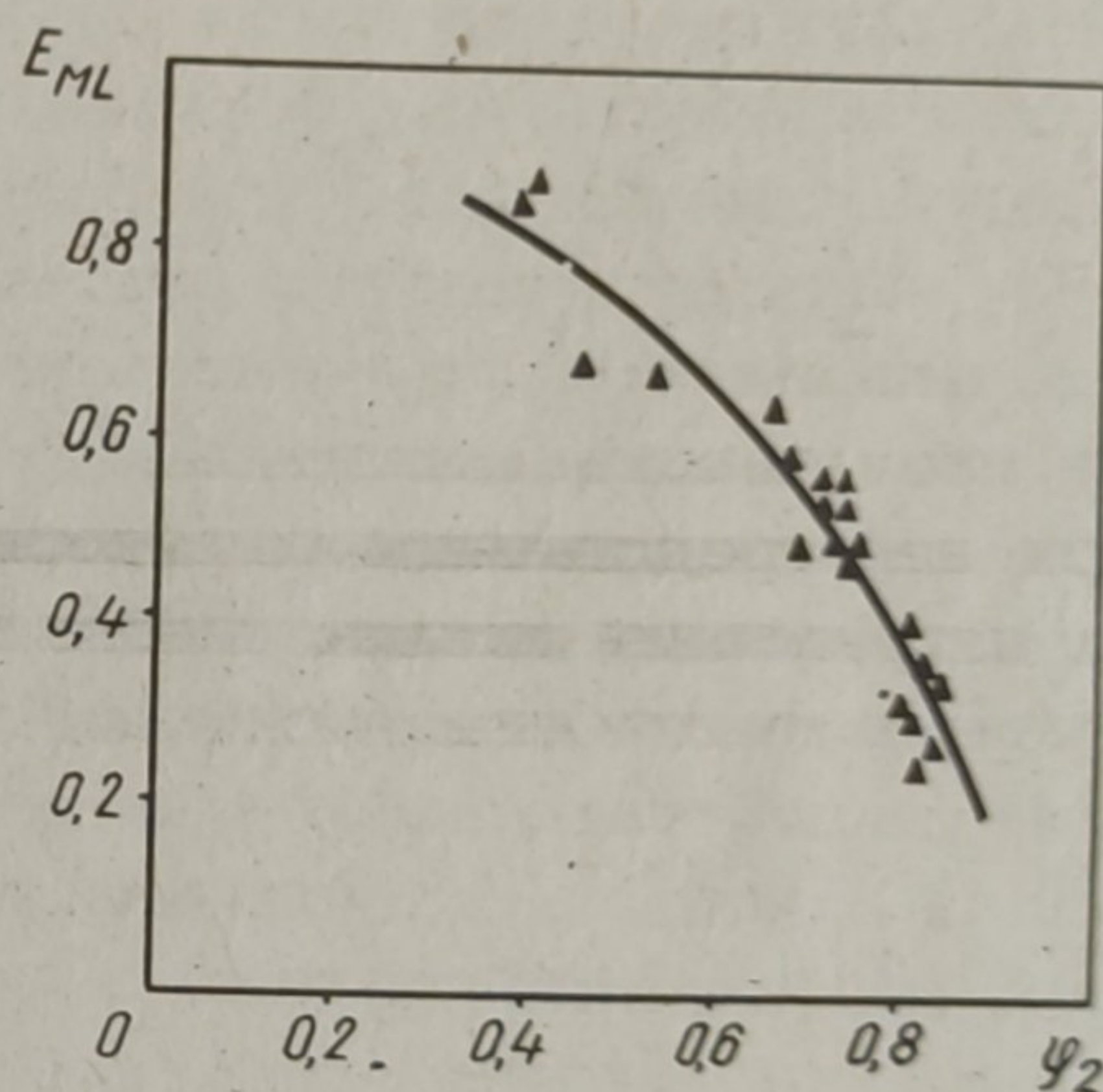
Рис. 2. Зависимость эффективности тарелки от доли байпасирующей жидкости
