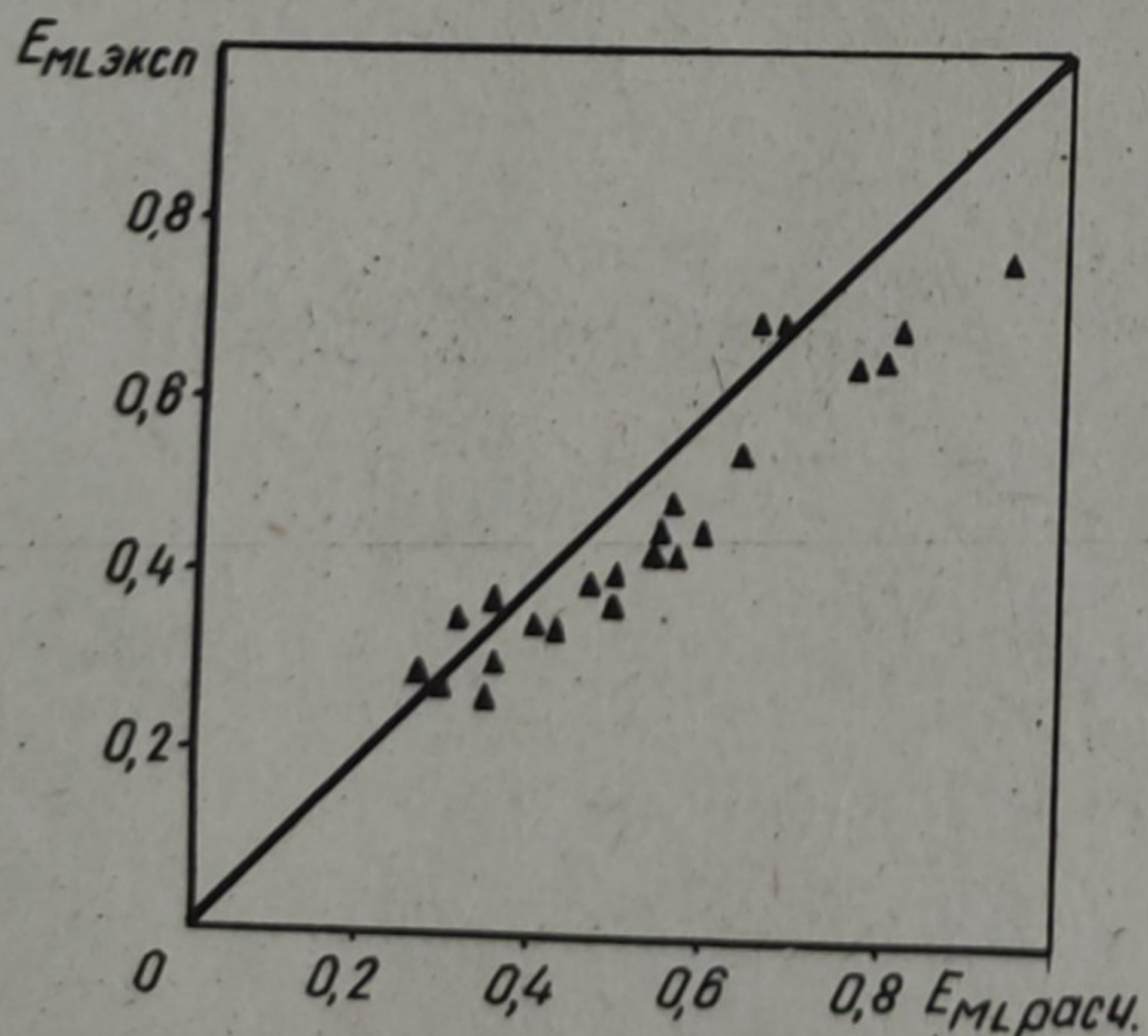
Рис. 1. Сравнение расчетных и экспериментальных значений эффективности тарелки
