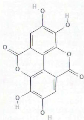
Эллаговая кислота
