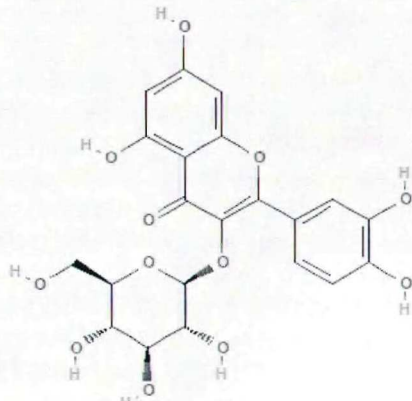
Кверцетин-3-О-гликозид
