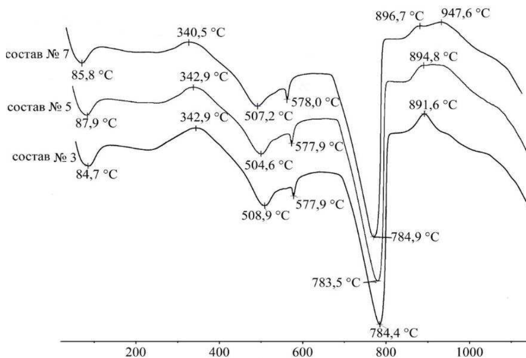
Рис. 2. Кривые ДСК исследованных шихт
