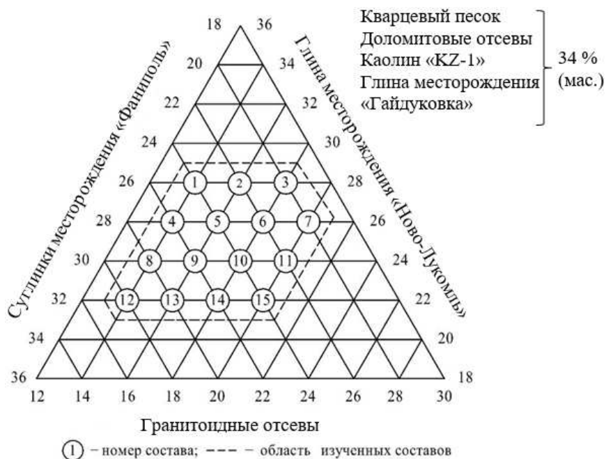
Рис. 1. Составы масс для керамических плиток внутренней облицовки стен
