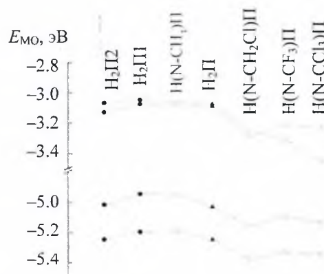
Рис. 6. Энергия четырех молекулярных орбиталей Гоутермана для исследуемых порфиринов
