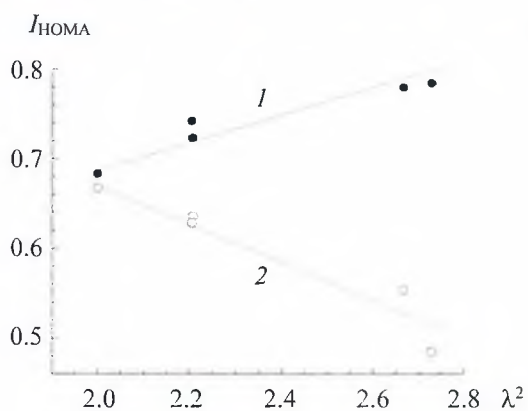
Рис. 3. Зависимость индекса ароматичности I_{НОМА} от степени гибридизации \lambda^2 атома азота замещенного пиррольного кольца: 18-членный аннуленоподобный контур (1), 22-членный контур Шлейера (2)
