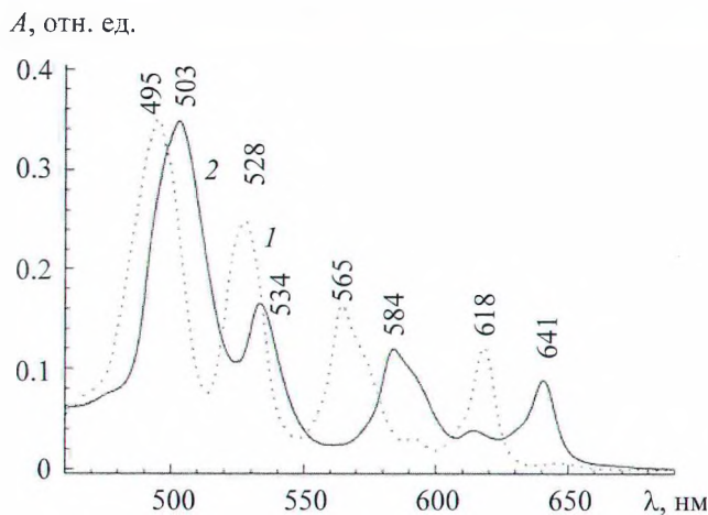
Рис. 1. Спектры поглощения в видимой области для 21,23- H,2,3,7,8,12,13,17,18 -октаэтилпорфирина ( H_2OЭП ) (1) и 21- CH_3,23-H,2,3,7,8,12,13,17,18 -октаэтилпорфирина ( H(N-CH_3)OЭП ) (2) в ацетонитриле
