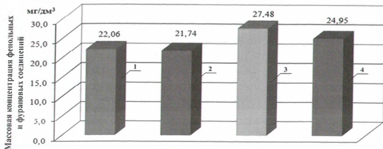
1 – образец № 1 - зерновой дистиллят, выдержанный в контакте с древесиной дуба отечественного происхождения при t=20 °С в течение 23 суток; 2 – образец № 2 - зерновой дистиллят, выдержанный в контакте с древесиной дуба иностранного происхождения при t=20 °С в течение 23 суток; 3 – образец № 3 - зерновой дистиллят, выдержанный в контакте с древесиной дуба отечественного происхождения при t=38 °С в течение 23 суток; 4 – образец № 4 - зерновой дистиллят, выдержанный в контакте с древесиной дуба иностранного происхождения при t=38 °С в течение 23 суток.
