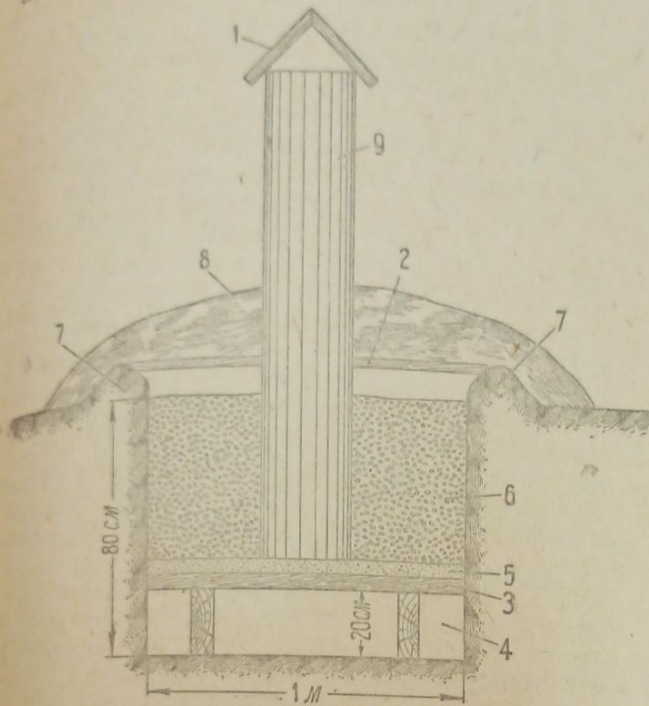
Рис. 1. Поперечный профиль теплой траншеи после засыпки семян осенью для подготовки к весеннему посеву:
