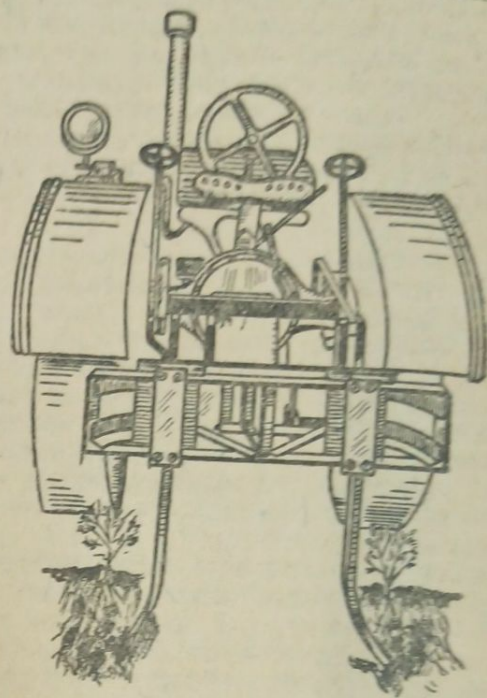
Рис. 2. Свеклоподъемник 3-НС
