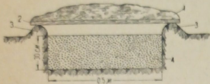
Рис. 3. Канавка для подготовки семян к позднему осеннему посеву:
