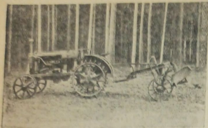
Рис. 2. Тракторный лесной плуг ТЛП ЦНИИЛХ в сцепке с трактором У-2
