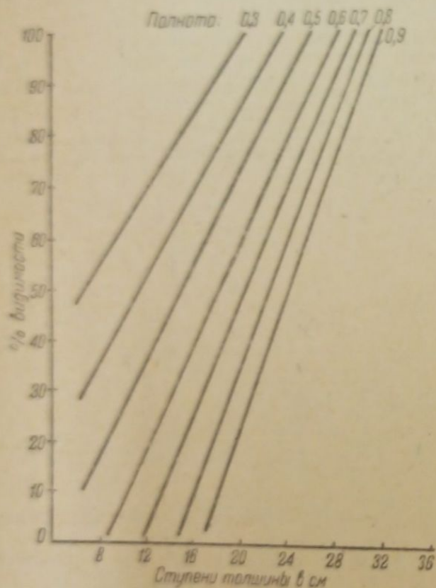
Рис. 1. Зависимость процента видимости ели первого и второго ярусов в спелых древостоях различной полноты с абсолютным преобладанием этой породы (масштаб снимков 1/10000 )
