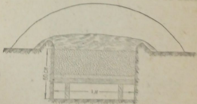
Рис. 2. Поперечный профиль холодной траншеи зимой после выпадения снега (верхний, незастратифицированный слой — снег; в случае малоснежной зимы насыпается слой 40—50 см)
