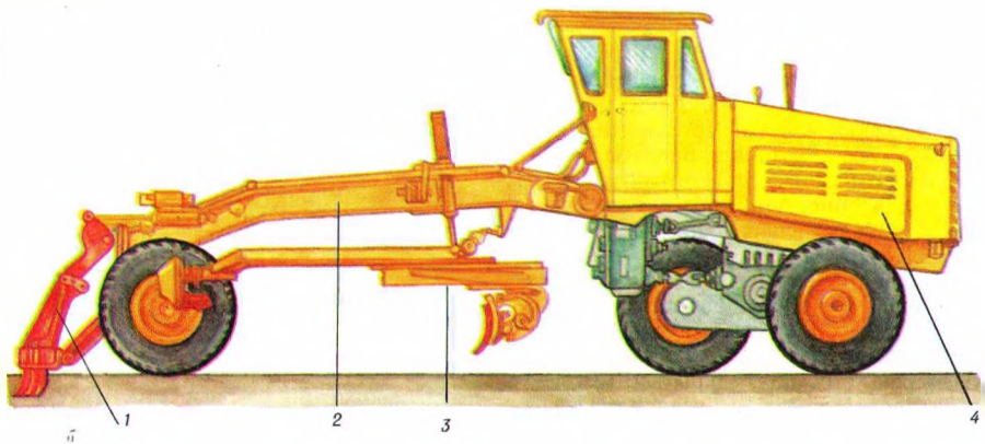
Грэйдэры: а — прычэпны (1 — механізм пад'ёму і апускання адвалу; 2, 3 — асноўная і цягавая рамы; 4 — адвал з нажом); б — аўтагрэйдэр (1 — кіркоўшчык; 2 — рулявы прывод; 3 — цягавая рама з паваротнымі кругамі і адвалам; 4 — рухавік з механізмамі кіравання).
