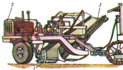
Паўпрычэпны грэйдэр-элеватар: 1 — нож; 2 — рухавік стужачнага транспарцёра; 3 — стужачны транспарцёр.
