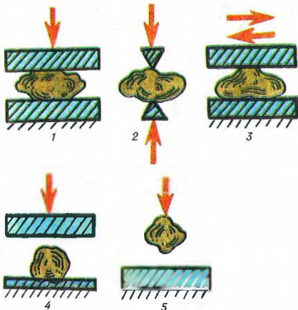
Спосабы драблення: 1 — расцісканне; 2 — расколванне; 3 — сціранне; 4, 5 — удары.
