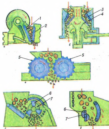
Схема драбілак: а — шчокавая (1, 2 — рухомая і нерухомае шчока); б — конусная (3, 4 — нерухомае і рухомыя конусы); в — валковая зубчастая (5 — валкі); з — малатковая (6 — малаток, 7 — ротар); д — ротарная.
