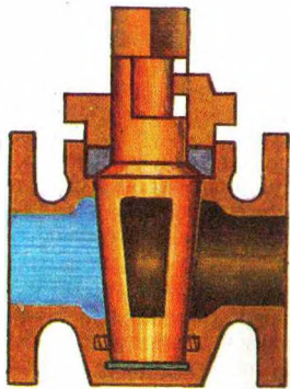
Праходны кран з прамалінейным рухам вадкасці.
