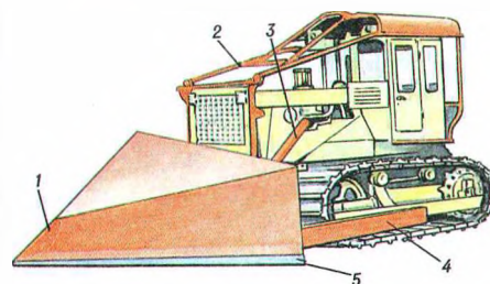
Кустарэз: 1 — адвал; 2 — агараджэнне трактара; 3 — гідрацыліндр; 4 — штурхальная рама; 5 — нож.
