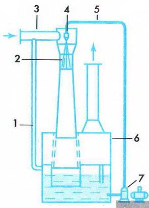
Схема скрубера: 1 — газаход; 2 — камера змешвання; 3 — прыёмны патрубак газу; 4 — фарсунка (распыляльнік вадкасці); 5 — трубаправод вадкасці; 6 — камера ачышчанага газу; 7 — помпа.
