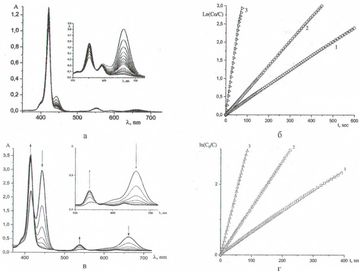
Рис. 3. (а) Изменение ЭСП (H 2 P3) в ходе реакции координации ацетатом цинка и (б) зависимость lgC 0 /C (1 – 291,15 К; 2 – 298,15 К; 3 – 308,15 К) (CH 2 P1 3·10 -5 моль/л, λ 680 нм, CZn(OAc) 2 1,34·10 -3 моль/л); (в) Изменение ЭСП (H 2 P3) в ходе реакции координации ацетатом меди и (г) зависимость lgC 0 /C (1 – 291,15 К; 2 – 298,15 К; 3 – 308,15 К) (CH 2 P1 3·10 -5 моль/л, λ 442 нм, CCu(OAc) 2 1,03·10 -3 моль/л)
