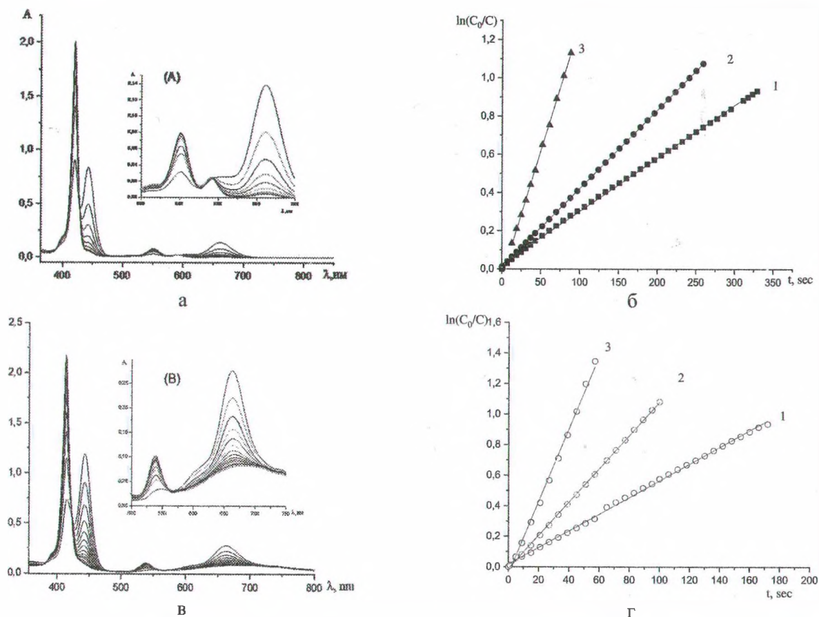
Рис. 5. (А) Изменение ЭСП ( H_2P_5 ) в ходе реакции координации ацетатом цинка и (Б) зависимость \lg C_0/C (1 – 291,15 К; 2 – 298,15 К; 3 – 308,15 К) ( CH_2P_1 1,82 \cdot 10^{-5} моль/л, \lambda 661 нм, CZn(OAc)_2 1,45 \cdot 10^{-3} моль/л); (В) Изменение ЭСП ( H_2P_5 ) в ходе реакции координации ацетатом меди и (Г) зависимость \lg C_0/C (1 – 291,15 К; 2 – 298,15 К; 3 – 308,15 К) ( CH_2P_1 1,82 \cdot 10^{-5} моль/л, \lambda 662 нм, CCu(OAc)_2 9,54 \cdot 10^{-4} моль/л)
