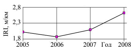
Рис. 1. Изменение ровности покрытия на участке автомобильной дороги М-4 км 49–53,3 в течение 2005–2008 гг. при уровне надежности 0,9
