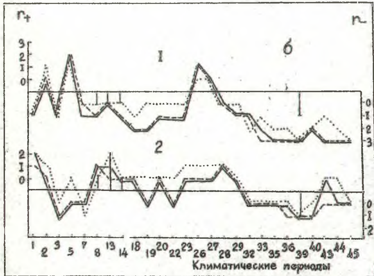
Рис. I. Корреляционные связи радиального прироста деревьев 2 пр.пл. (а) и 6 пр.пл. (б) в целом с климатическими периодами. 1 - с температурами, 2 - с осадками. - - - раннего, ..... позднего, ————— годовичного приростов. Вертикальными линиями показаны связи полученные по данным других авторов
