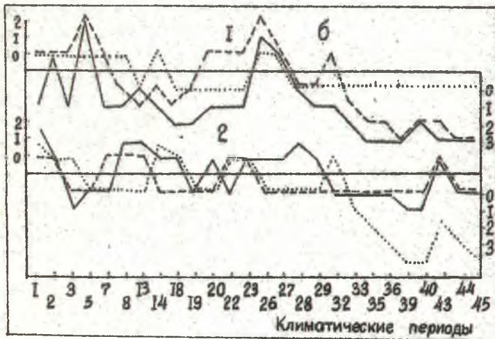
Рис.2. Корреляционные связи радиального прироста на отдельных пробных площадях в целом с климатическими периодами. а - нормальные местопрорастания (по раннему приросту), б - болотные (по годовичному приросту). 1 - с температурами, 2 - с осадками. — 1; 6 пр.пл., - - - 2; 7 пр.пл., ..... 3; 8 пр.пл., -.-.-.- 4 пр.пл.
