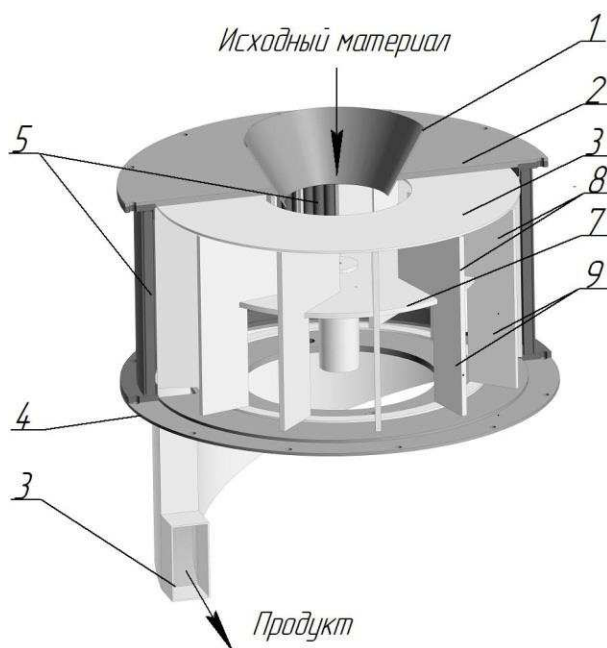
Рисунок 1 – Устройство ударно-центробежной мельницы
