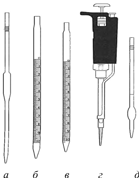
Рис. 4.2. Пипетки:
