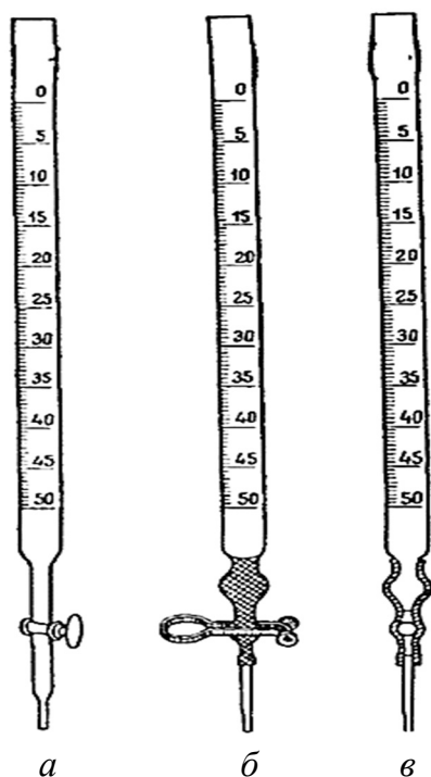
Рис. 4.3. Бюретки:
