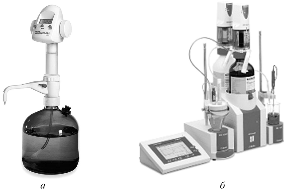
Рис. 4.5. Современное оборудование для титрования: а – цифровая бутылочная бюретка; б – автоматический титратор
