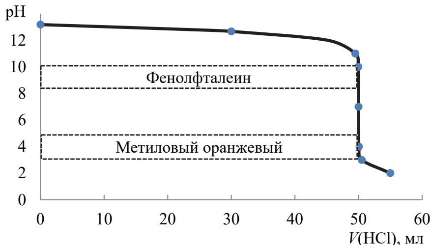
Рис. 5.5. Кривая титрования 100 мл 0,15 н. раствора NaOH 0,30 н. раствором HCl (построена с учетом разбавления раствора в процессе титрования)
