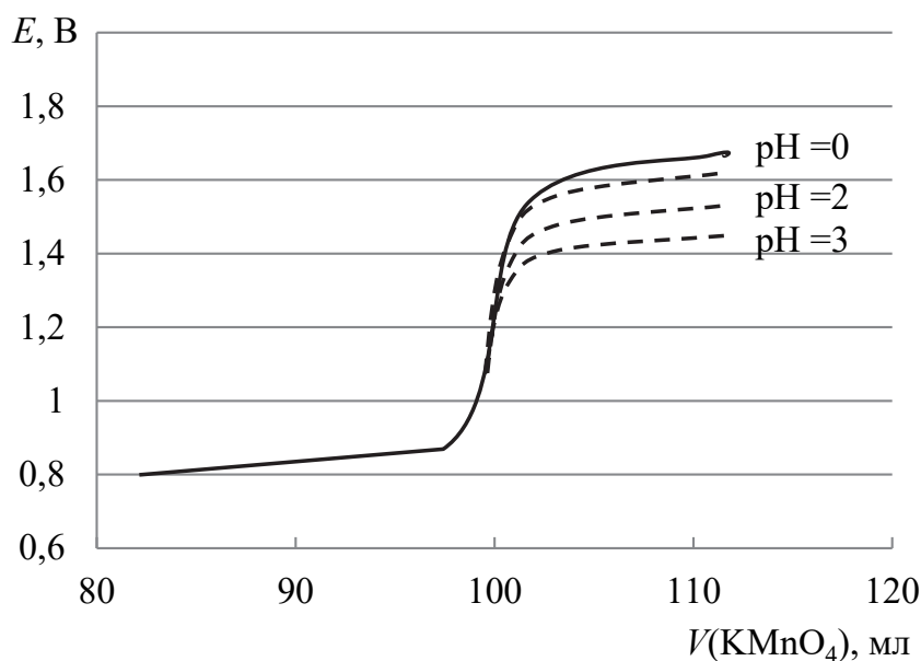
Рис. 6.2. Кривые титрования раствора Fe^{2+} раствором KMnO_4 при различных значениях pH раствора
