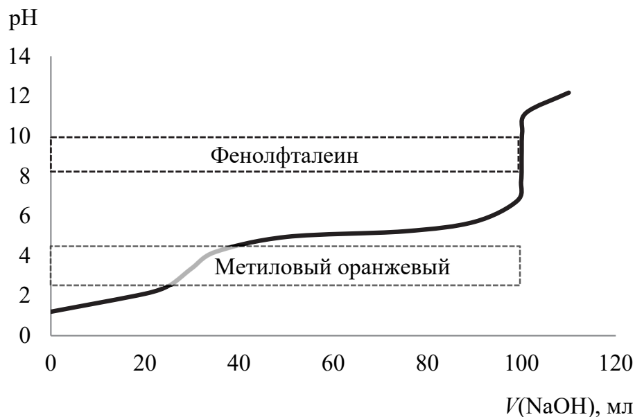
Рис. 5.4. Кривая титрования смеси \text{HCl} и \text{CH}_3\text{COOH}
