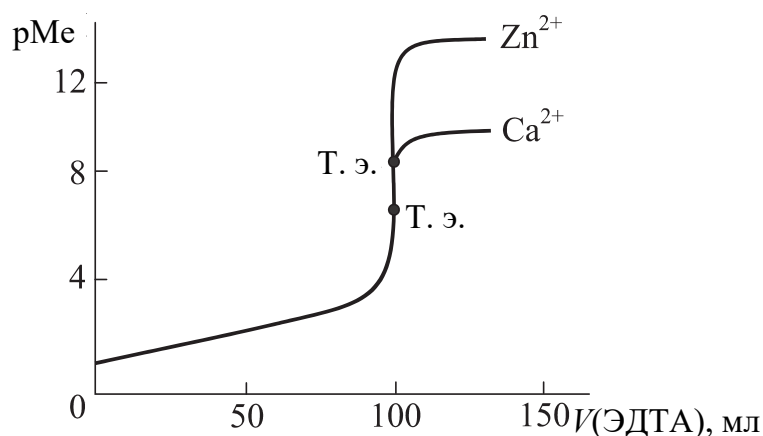
Рис. 7.3. Влияние константы устойчивости комплексоната на величину скачка: для \text{Ca}^{2+} \lg K = 10,59 ; для \text{Zn}^{2+} \lg K = 16,26
