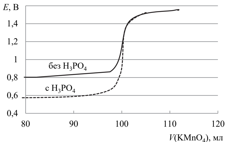
Рис. 6.3. Влияние \text{H}_3\text{PO}_4 на величину скачка кривой титрования раствора \text{Fe}^{2+} раствором \text{KMnO}_4
