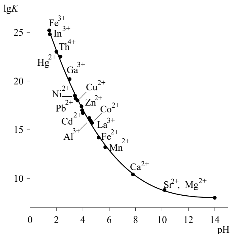
Рис. 7.1. Минимальное значение pH, необходимое для удовлетворительного титрования ионов металлов
