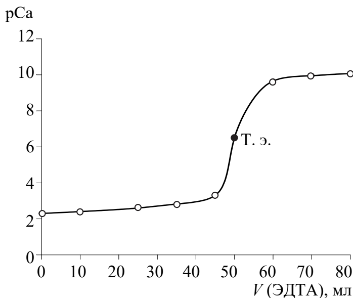
Рис. 7.2. Кривая титрования 0,025 моль/л раствора Ca^{2+} 0,025 моль/л раствором Y^{4-} при pH = 11 (построена с учетом разбавления раствора при титровании)
