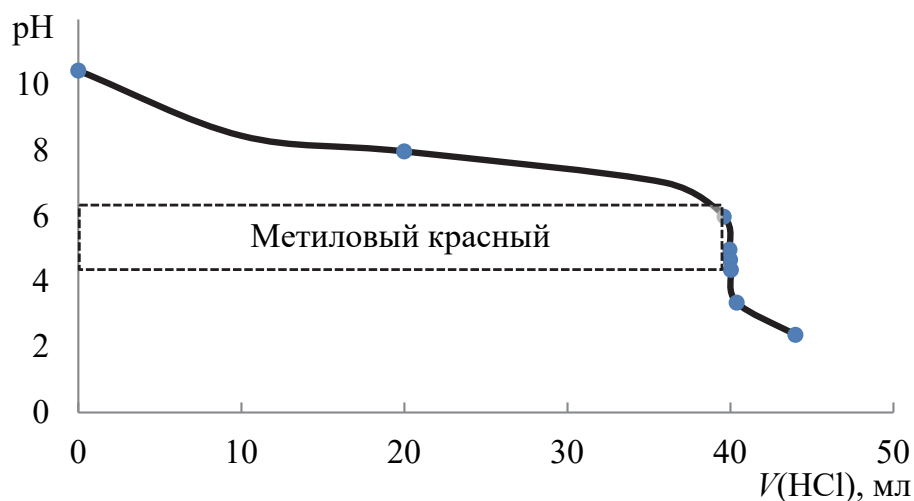
Рис. 5.6. Кривая титрования 50 мл 0,08 н. раствора \text{N}_2\text{H}_5\text{OH} 0,1 н. раствором HCl (построена с учетом разбавления раствора при титровании)
