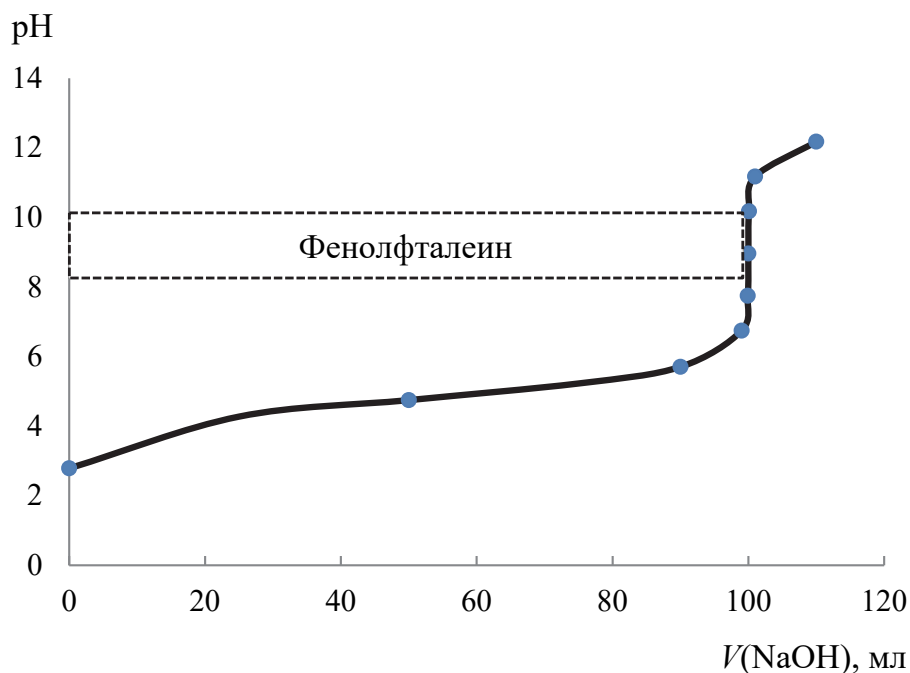
Рис. 5.2. Кривая титрования 100 мл 0,15 н. раствора CH 3 COOH 0,15 н. раствором NaOH (построена без учета разбавления раствора при титровании)
