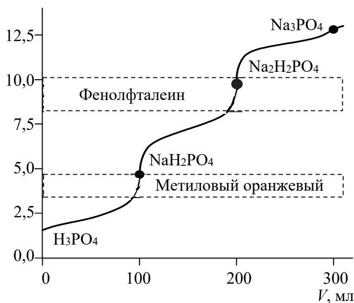
Рис. 5.3. Кривая титрования \text{H}_3\text{PO}_4 раствором \text{NaOH}
