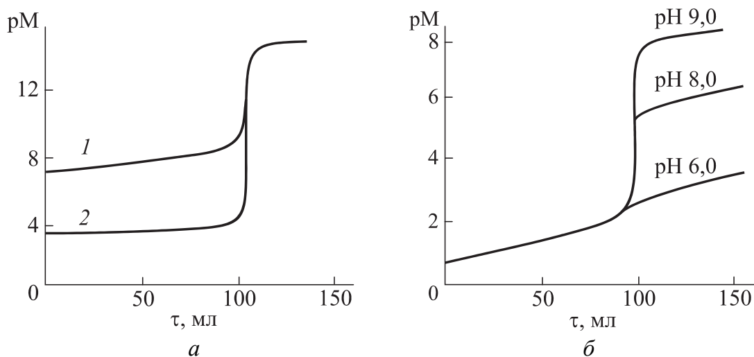
Рис. 7.4. Влияние побочных реакций по металлу (а) и по лиганду (б) на величину скачка:
