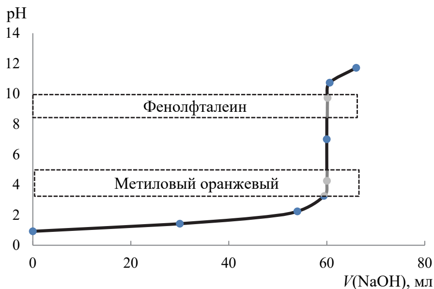
Рис. 5.1. Кривая титрования 50 мл 0,12 н. раствора HCl 0,1 н. раствором NaOH (построена с учетом разбавления раствора при титровании)
