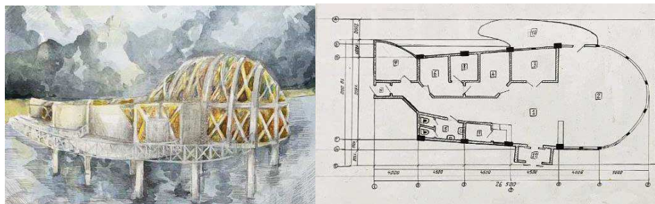
а) перспектива б) план Рисунок – Павильон рыбацкого клуба (Зеленкевич В.В.)
