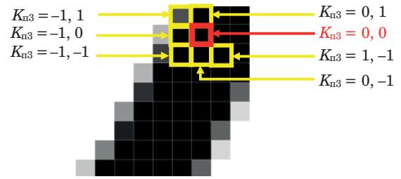
■ Рис. 2. Относительное пространственное положение пикселя в зависимости от ключа K_{\Pi 3}
