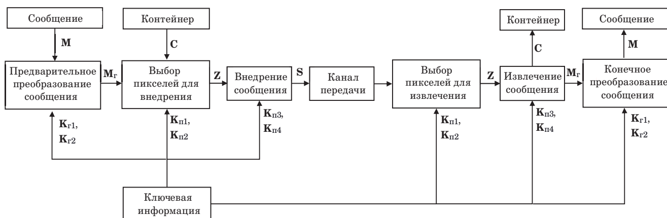
■ Рис. 3. Структурная схема описанной стеганографической системы
