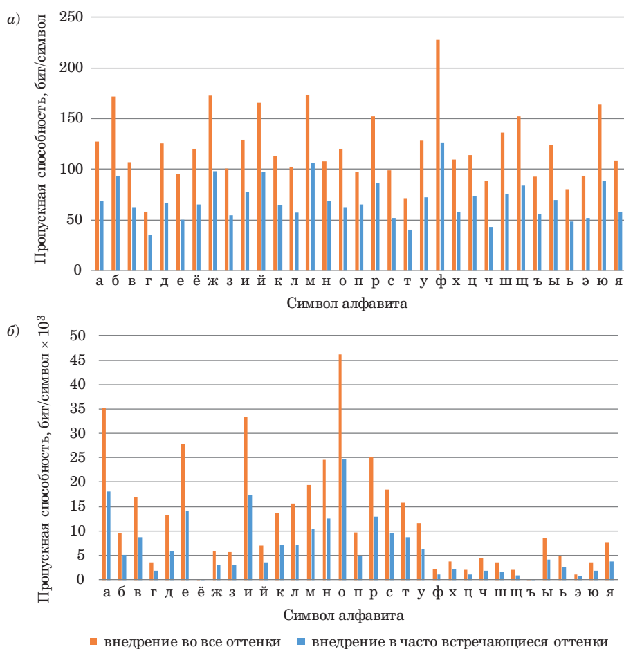
■ Рис. 8. Пропускная способность одного символа растрованного текста (а) и символов текста-контейнера (б) ■ Fig. 8. Bandwidth of one symbol of rasterized text (a) and of text of text-container (b)
