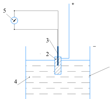
Рис. 2. Схема измерения температуры:
