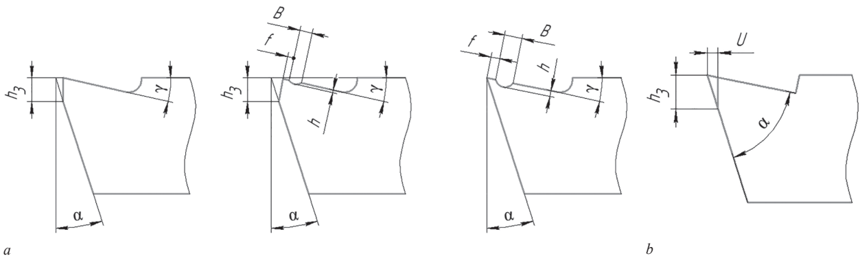
Рисунок 1 — Износ реза: а — виды износа; б — параметры износа Figure 1 — Cutter wear: а — wear types; б — wear parameters
