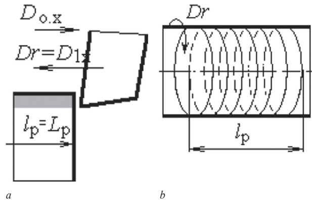
Рисунок 2 — Длина l_p и путь L_p резания при обработке: а — с прямолинейной формой главного движения; б — с круговой формой главного движения (путь резания показан тонкой линией) Figure 2 — Cutting length l_p and path L_p during processing: а — with a straight-linear mode of the main motion; б — with a circular mode of the main motion (the cutting path is shown as a thin line)
