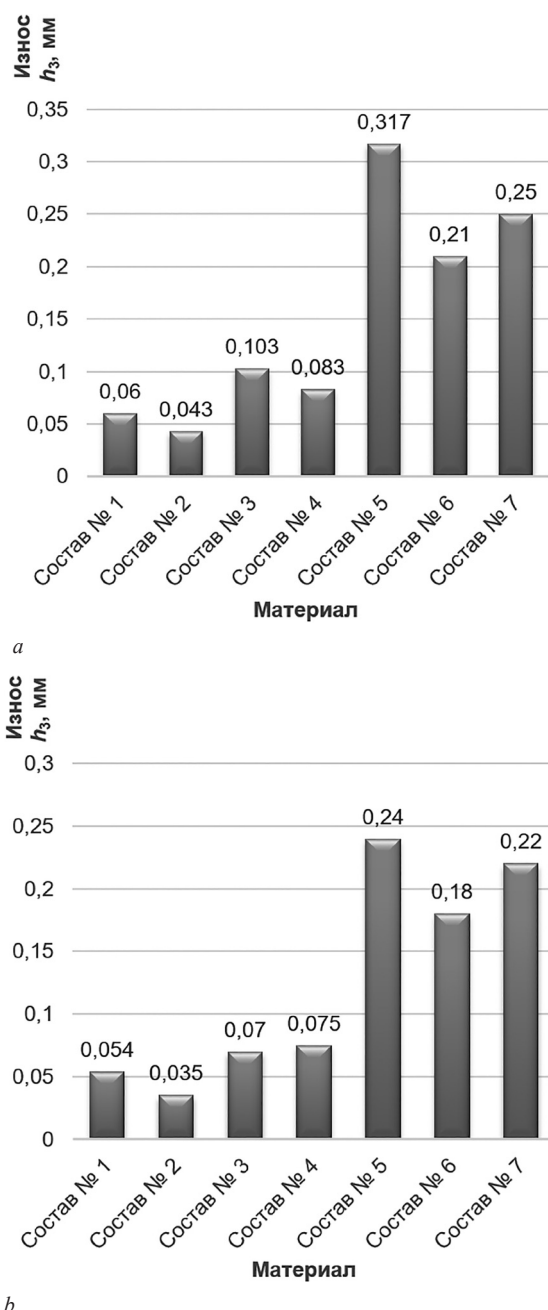
Рисунок 5 — Результаты испытаний металлообрабатывающих инструментов по критерию площадки износа: a — обработка алюминиевого сплава АК-7; b — обработка латуни ЛС 59-1 Figure 5 — Results of tests of metalworking tools according to the criterion of wear area: a — АК-7 aluminum alloy processing; b — LS 59-1 brass processing
