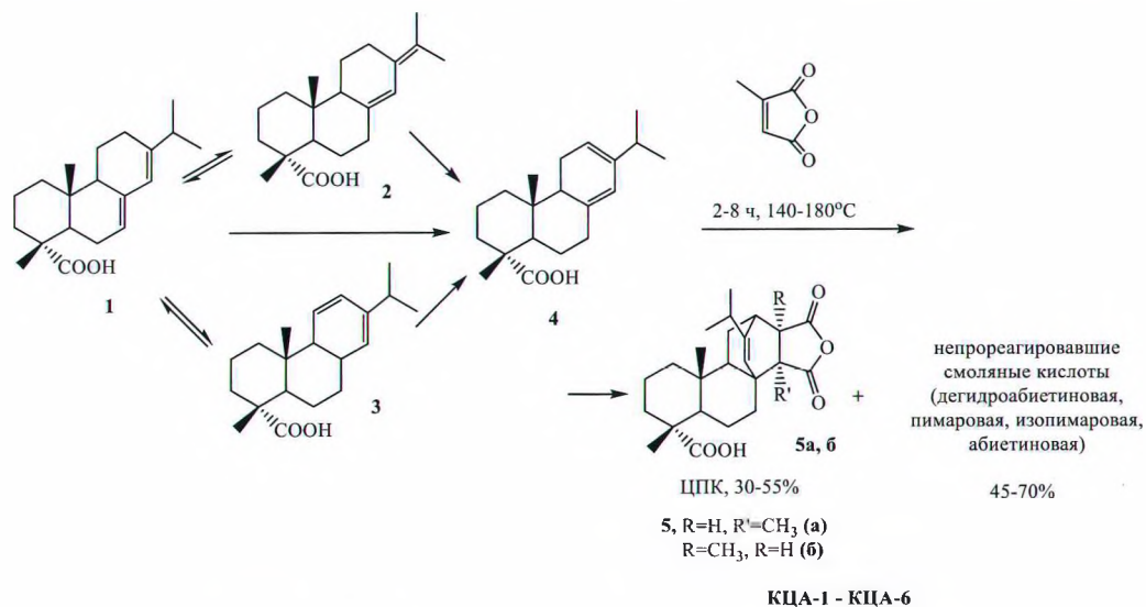
Рис. 1. Получение канифольноцитраконовых аддуктов КЦА-1–КЦА-6
