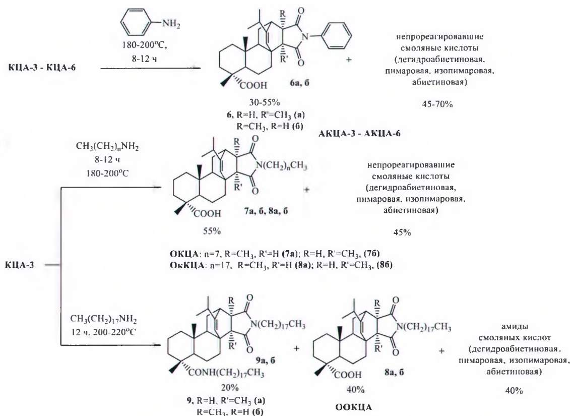
Рис. 2. Получение азотсодержащих производных канифольноцитраконовых аддуктов АКЦА-3 – АКЦА-6, ОКЦА, ОкКЦА, ООКЦА
