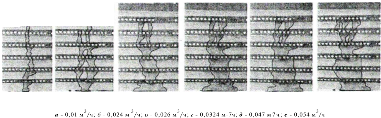
Рисунок 8. - Пленочное течение на гофрированном листе с перфорацией (оборотная сторона) и длиной образующей 8 мм
