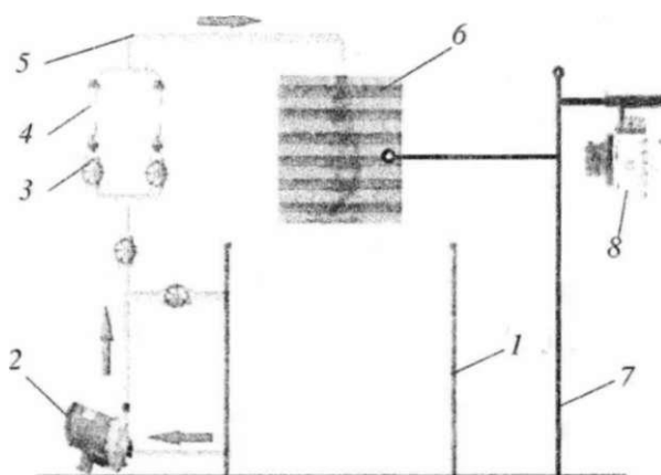
1 - резервуар; 2 - центробежный насос; 3 - вентиль; 4 - ротаметр; 5 - трубопроводная система; 6 - гофрированный лист; 7 - штатив; 8 - камера
