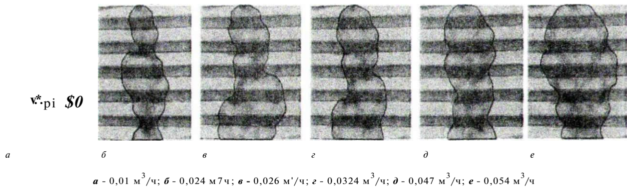
Рисунок 9. - Пленочное течение на гофрированном листе без перфорации и длиной образующей 11 мм
