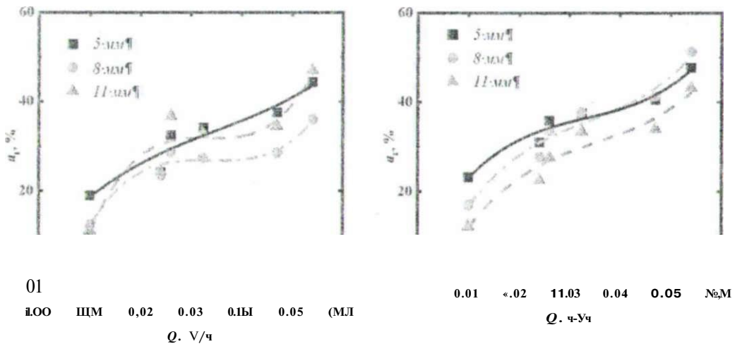
Рисунок 11. - Изменение удельной величины смоченной поверхности <math>a_r</math> от расхода жидкости Q , м³/ч, для гофрированных листов
