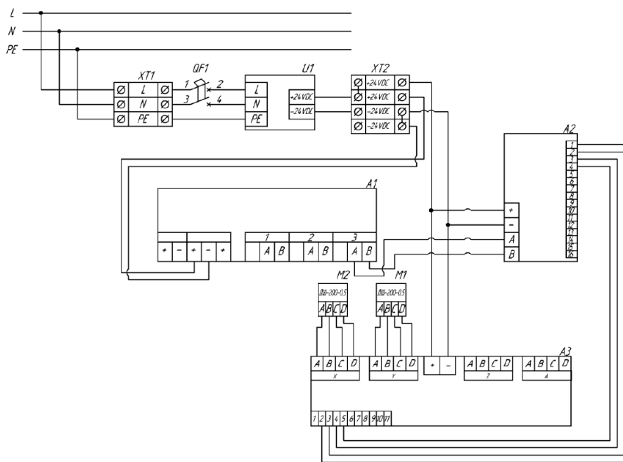
Рисунок 3 – Электрическая схема подключений системы
